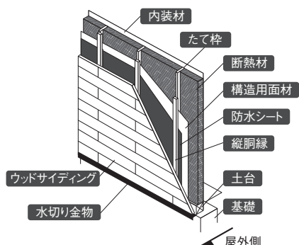
枠組壁工法 横貼り(T&G・ペネル)
