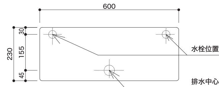
開口寸法
