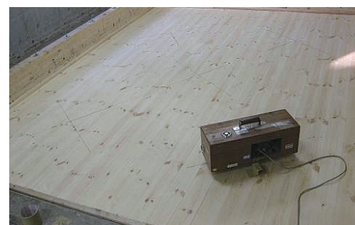
軽量床衝撃音試験（タッピングマシン）
