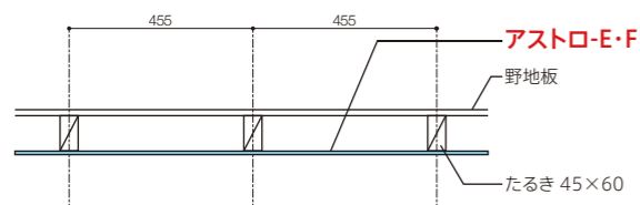
○たるき間隔 455mm たるき 45x60mm
