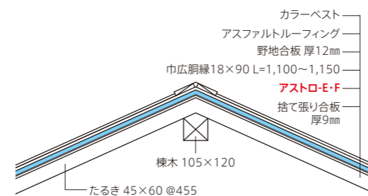
スレート参考施工図
