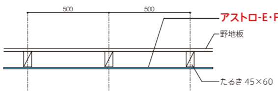
○たるき間隔 500mm たるき 45x60mm
